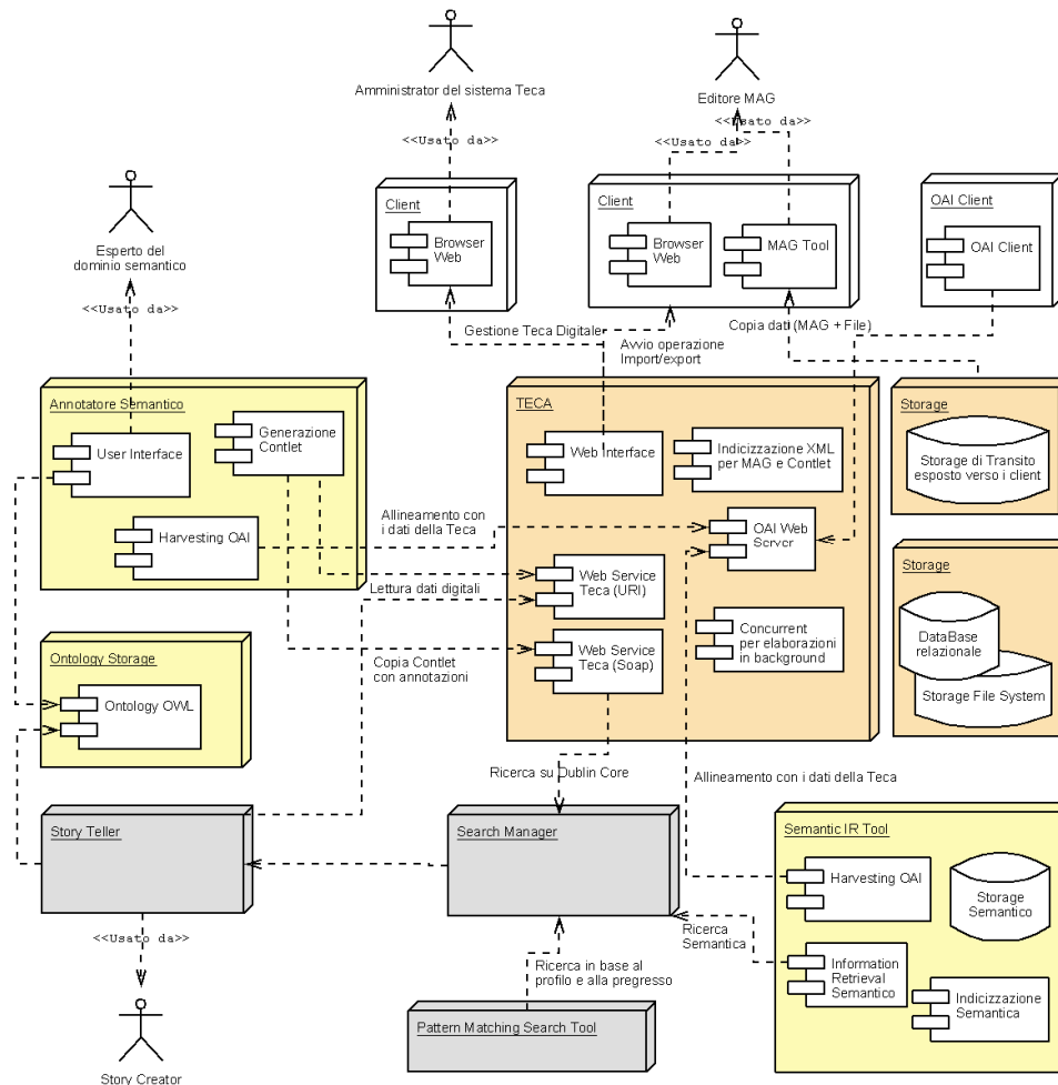
Figura 1 – Diagramma di deployment del MAG-Repository
