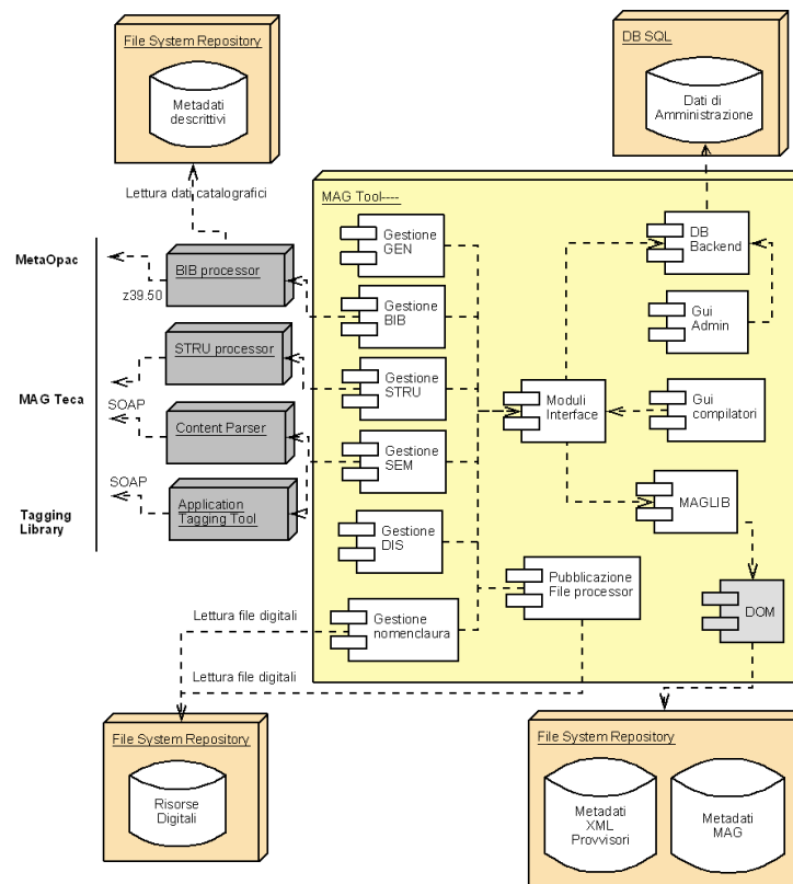
Figura 1 – Diagramma di deployment del MAGTool
